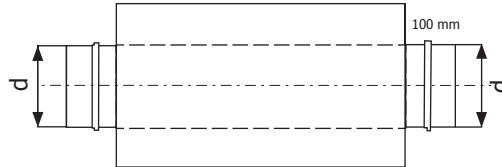
Tlumič hluku kruhový TH/100
