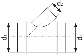
Odbočka jednostranná 45°
