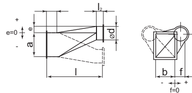
KOLENO, KOLENO PŘECHODOVÉ symetrický nebo asymetrický; R_{\min}=100 mm
