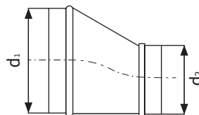
Přechod asymetrický
