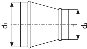
Přechod osový
