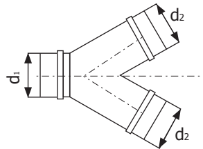
Rozbočka symetrická 60°
