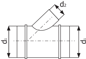
Odbočka jednostranná 45°
