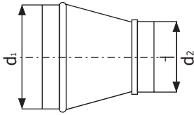
Přechod osový
