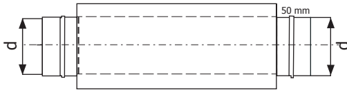
Tlumič hluku kruhový TH/50
