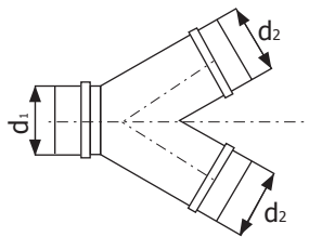
Rozbočka symetrická 60°
