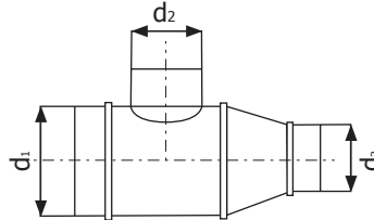
Odbočka přechodová 90°
