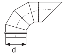
Oblouk segmentový výfukový 90° (VOBL)
