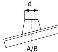
Střešní průchod 5° - 27° (PS5-27)
