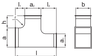
ROZBOČKA SYMETRICKÁ symetrická a=a^1 ; R_{\min}=100 mm
