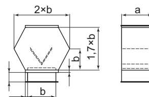
VÝFUKOVÁ HLAVICE se sítí proti vniknutí drobných částic
