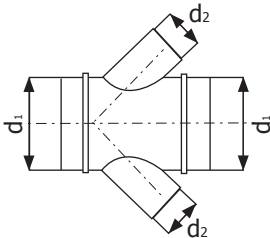
Odbočka oboustranná 45°
