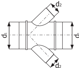
Odbočka oboustranná 45°
